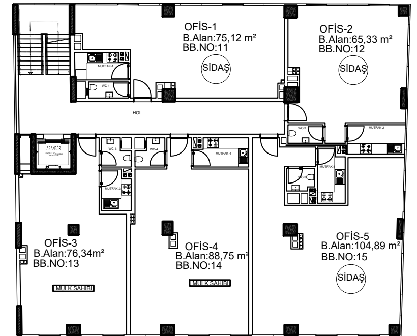
3.NORMAL KAT PLANI
